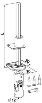
D845 NG BLANC H7RONDE DE 12 L320
