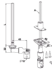
D776NG M.B.G D22AL 12-6P7 L175 BLANC
