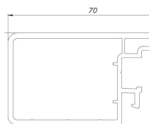
SUPPORT DE GALET HAUT EASYCLICK 200
