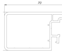
SUPPORT DE GALET HAUT EASYCLICK 200
