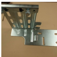
PLAQUE AVANT EASYCLICK 200 DROITE RENFORCEE
