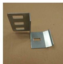
PROFIL DE FIXATION GABARIT GAUCHE
